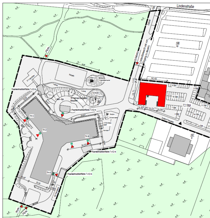
Lageplan Container M 1:1000
