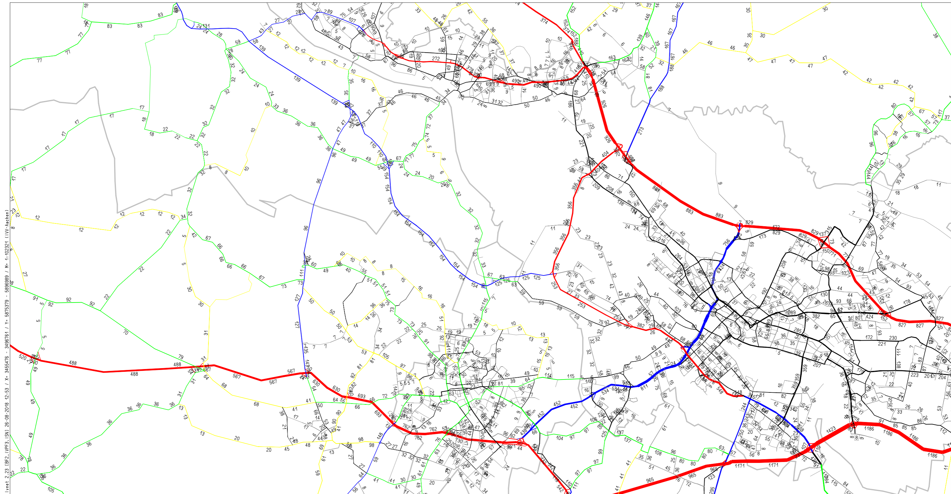
BF2 - VU B 212n. Planfall 3 B 212n 2030; Kfz-Belastungen am mittleren Werktag [Kfz/Tag] (Stand: 24.08.2018) (in 100er, ohne Werte < 500)
