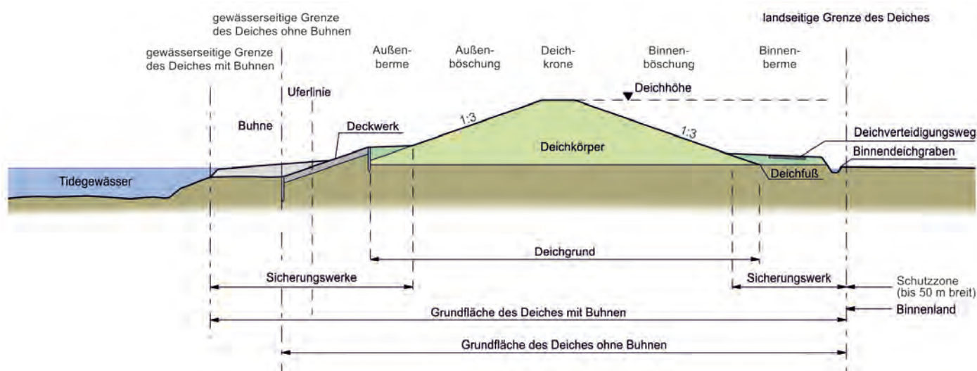
Abb. 6-3: Regelquerschnitt eines scharliegenden Schutzdeiches
